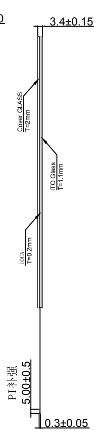
侧视图
