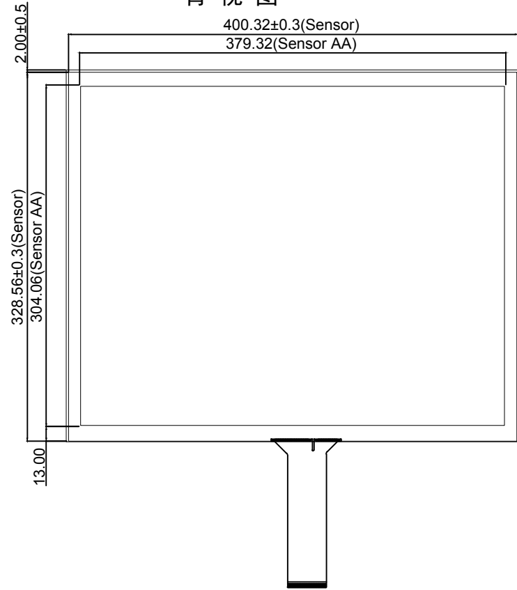
背视图
