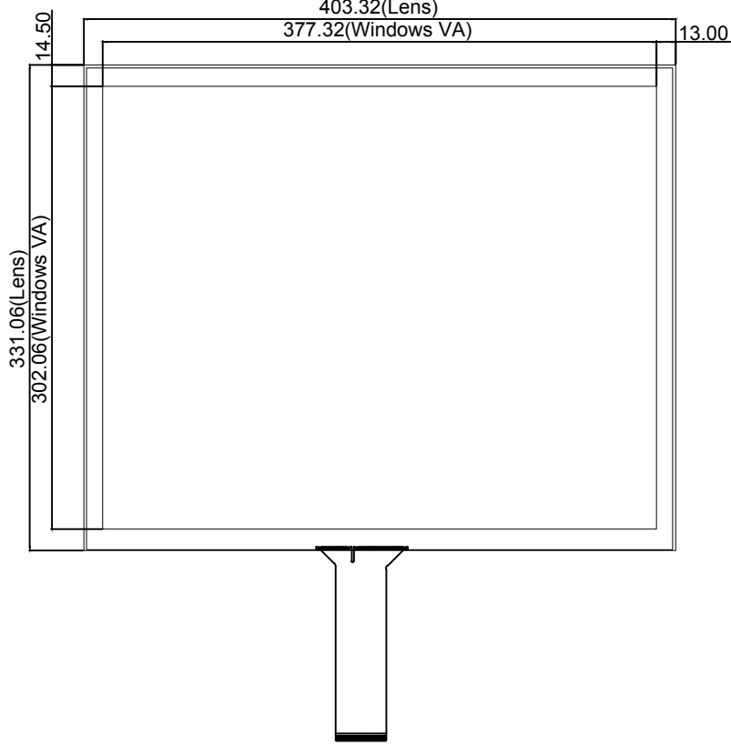
正视图
