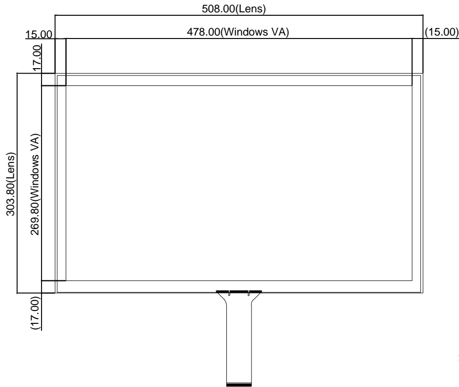
正视图
